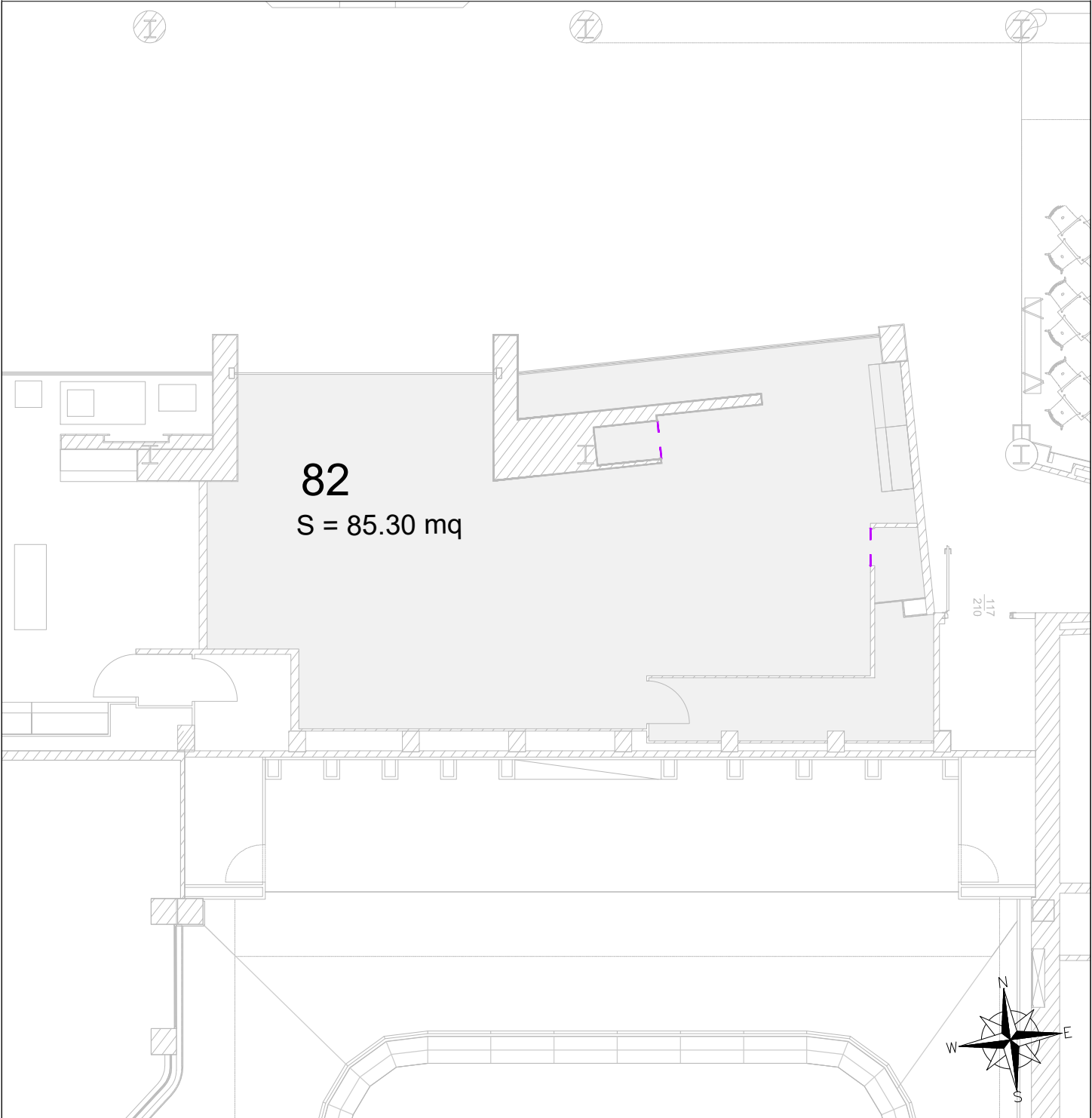
PIANTA scala 1:100
