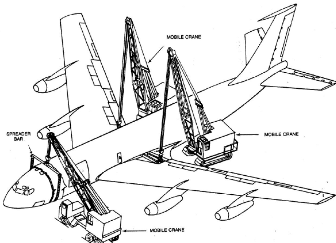
Fig. 3 Esempio di sollevamento dell'intero aeromobile tramite gru mobili
